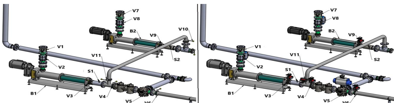
FIGURA 1. Desenho técnico do sistema atual para o automatizado.
