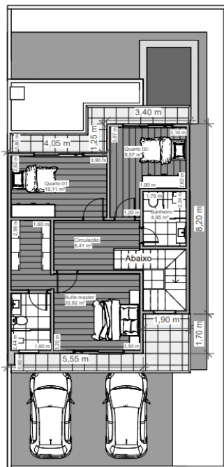
FIGURA 2. Planta baixa do segundo pavimento.
