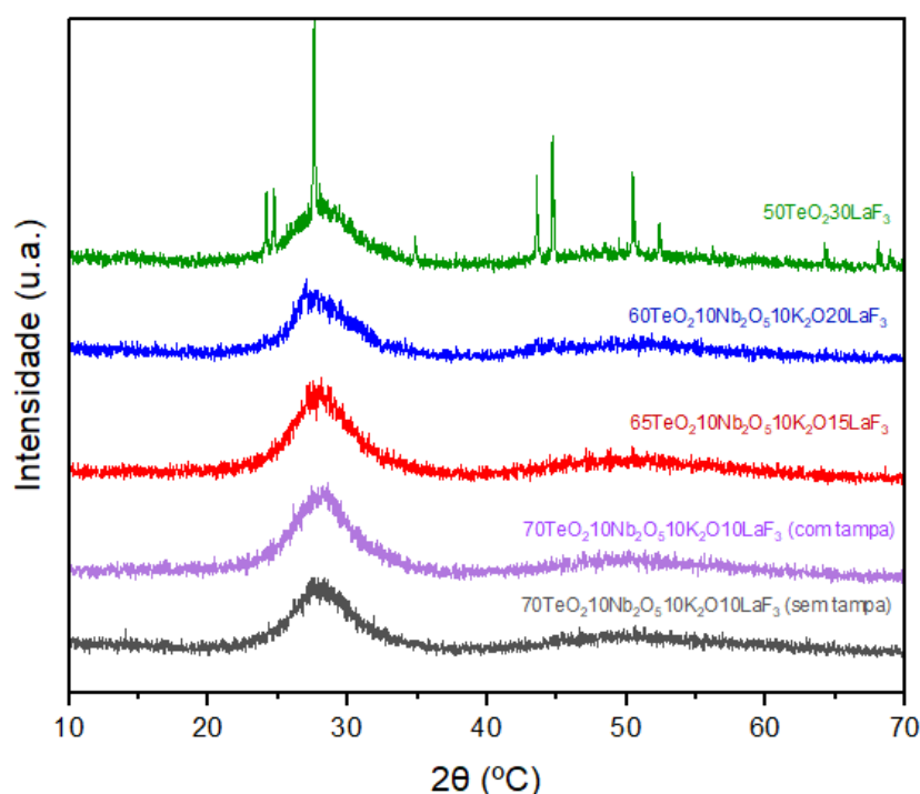
FIGURA 2. Padrões de difração de raios-X (DRX) para diferentes composições de vidros no sistema \text{TeO}_2\text{-Nb}_2\text{O}_5\text{-K}_2\text{O-LaF}_3 em diversas condições de processamento e concentrações de \text{LaF}_3 .
