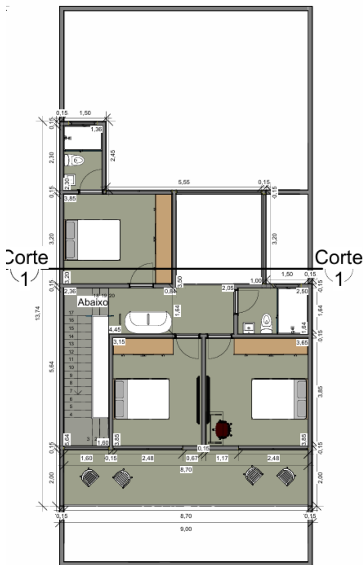
FIGURA 3. Planta Baixa do Segundo Pavimento.
