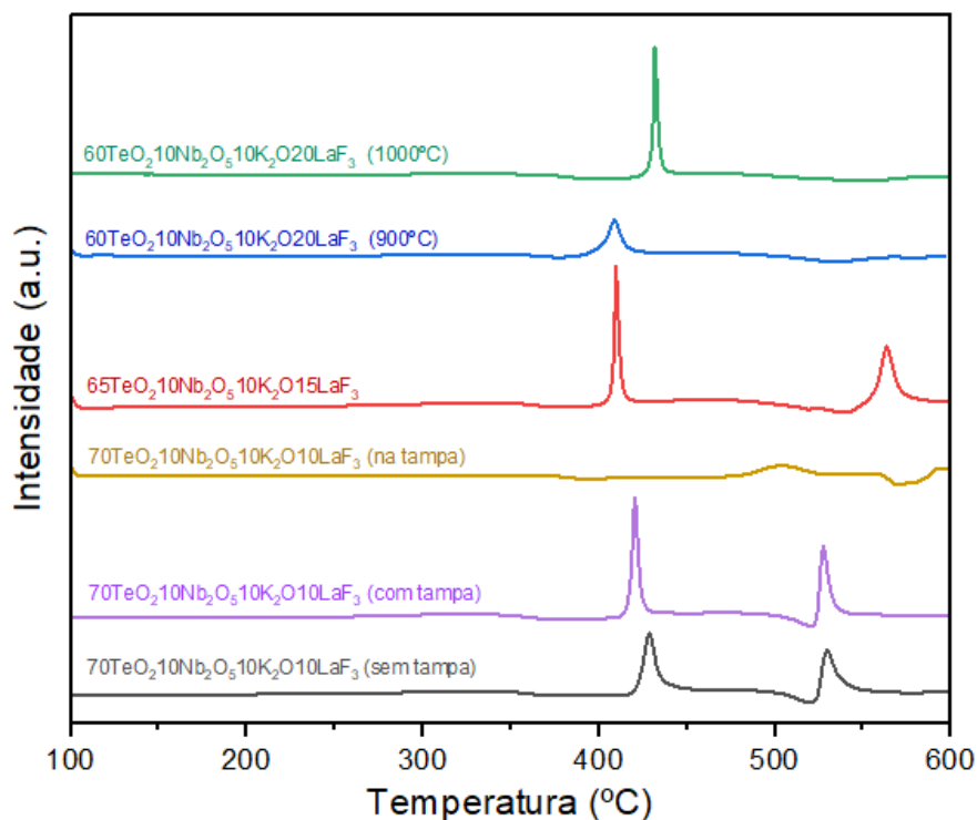
FIGURA 1. Curvas de DSC para diferentes composições de vidros no sistema \text{TeO}_2\text{-Nb}_2\text{O}_5\text{-K}_2\text{O-LaF}_3 .
