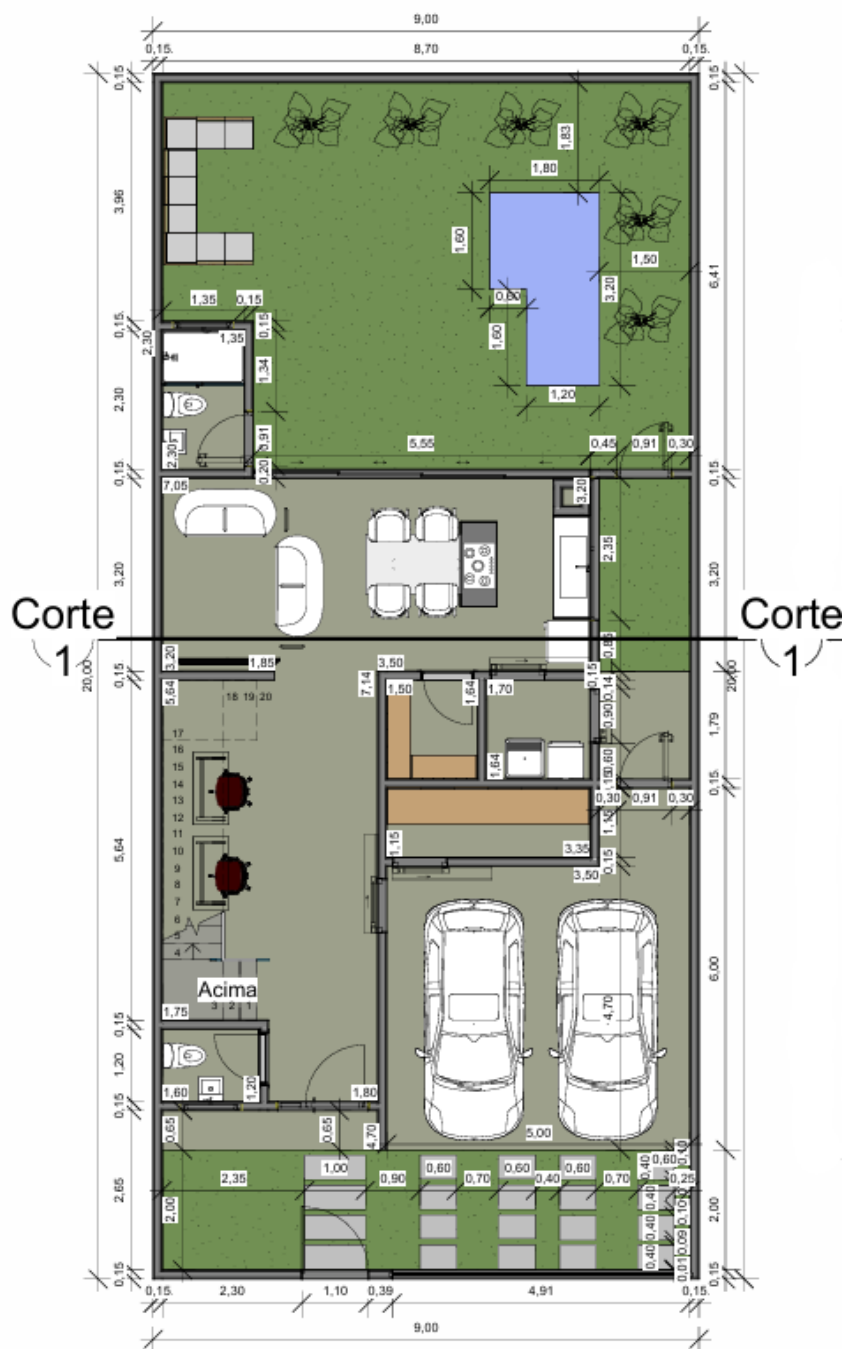
FIGURA 2. Planta Baixa do Pavimento Térreo.
