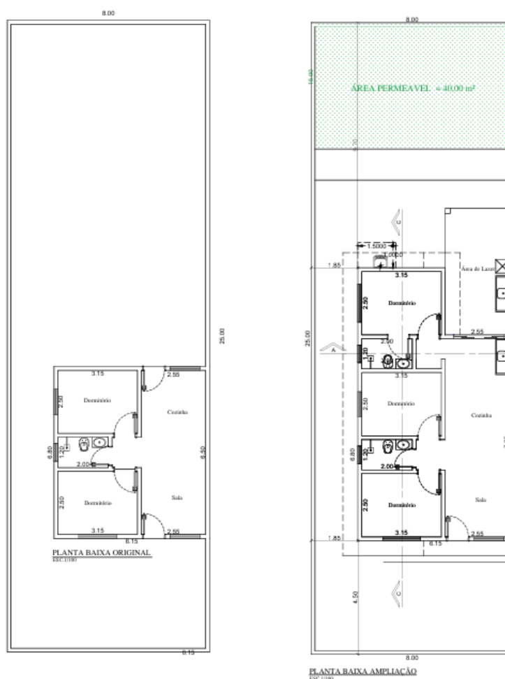
FIGURA 2. Reprodução em AutoCad de planta baixa disponibilizada em sala de aula e ampliação proposta.
