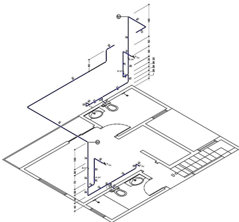
FIGURA 9. Planta Isométrica Hidrossanitário Água Fria. FONTE: José Walter, 2024.
