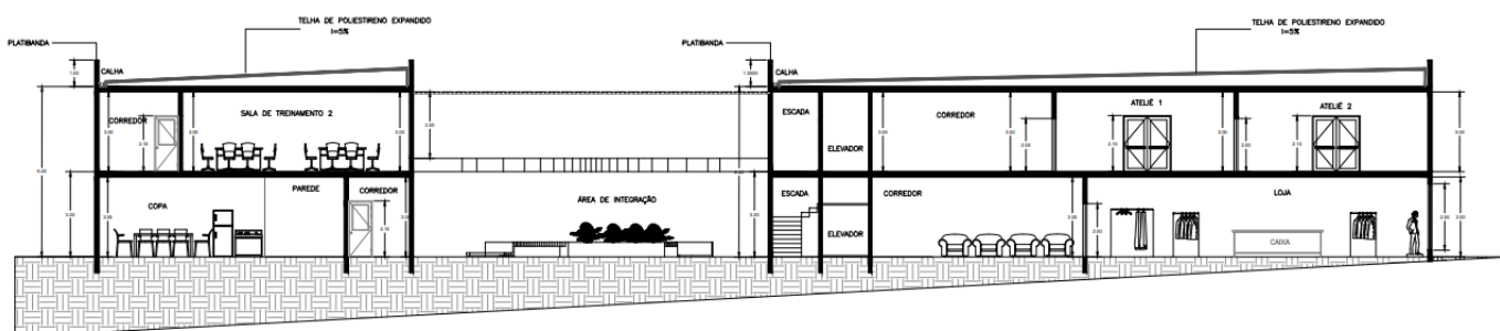
FIGURA 9. Corte AA do Projeto Costurando Sonhos Brasil.
