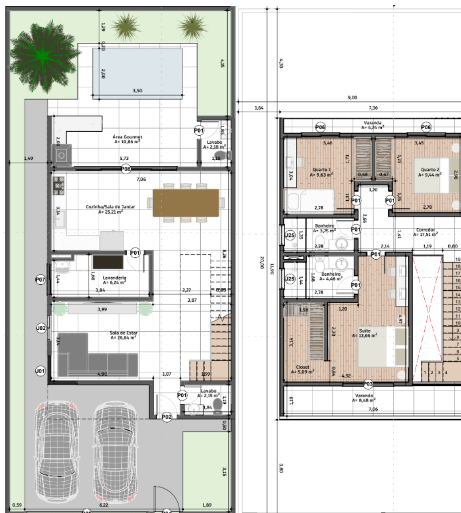
FIGURA 3. Projeto arquitetônico, sem escala.
