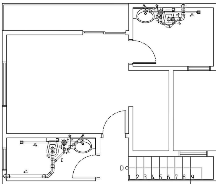
FIGURA 10. Planta Hidrossanitária Esgoto Pavimento Superior FONTE: José Walter, 2024.
