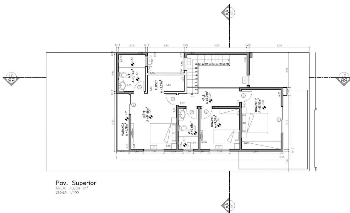
FIGURA 2. Planta Baixa Pavimento Superior.
