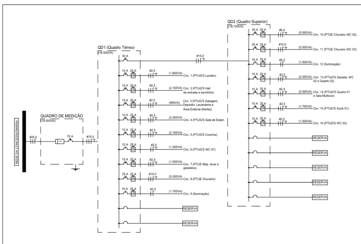
FIGURA 5. Diagrama Multifilar.
