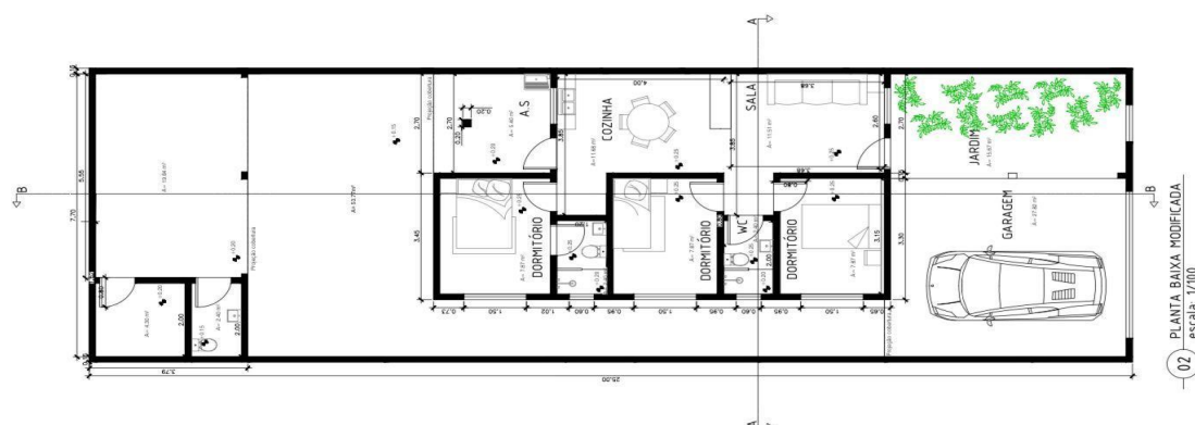
FIGURA 2. Planta baixa de ampliação.
