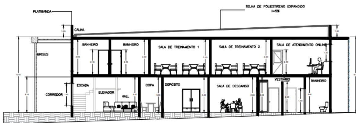
FIGURA 10. Corte BB do Projeto Costurando Sonhos Brasil.
