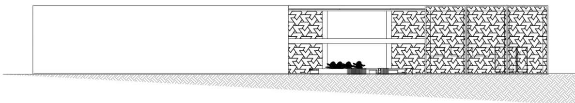
FIGURA 7. Elevação 3 do Projeto Costurando Sonhos Brasil.
