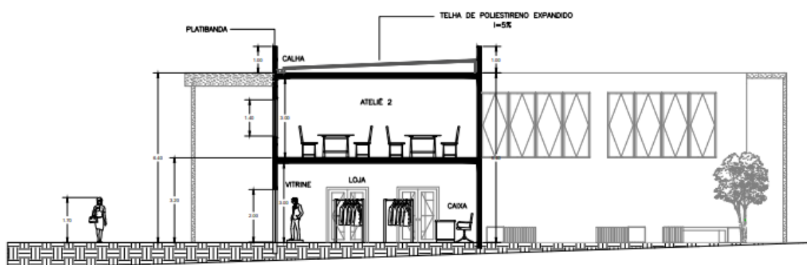
FIGURA 11. Corte CC do Projeto Costurando Sonhos Brasil.
