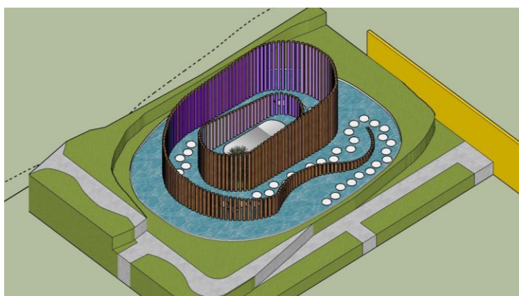
IMAGEM 3. Perspectiva frontal da folie , feita no SketchUp.
