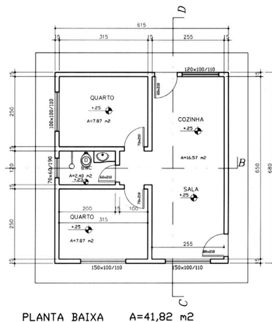
FIGURA 1. Planta baixa original
