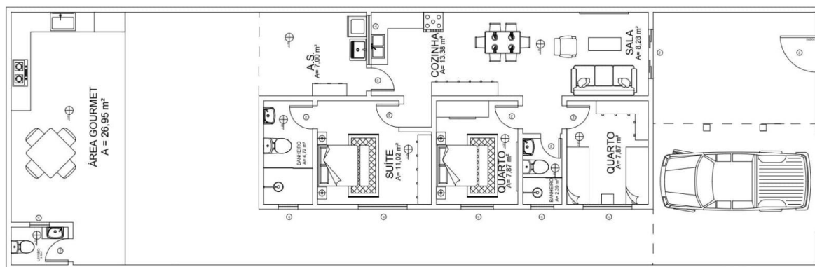
FIGURA 2. Planta baixa ampliada.
