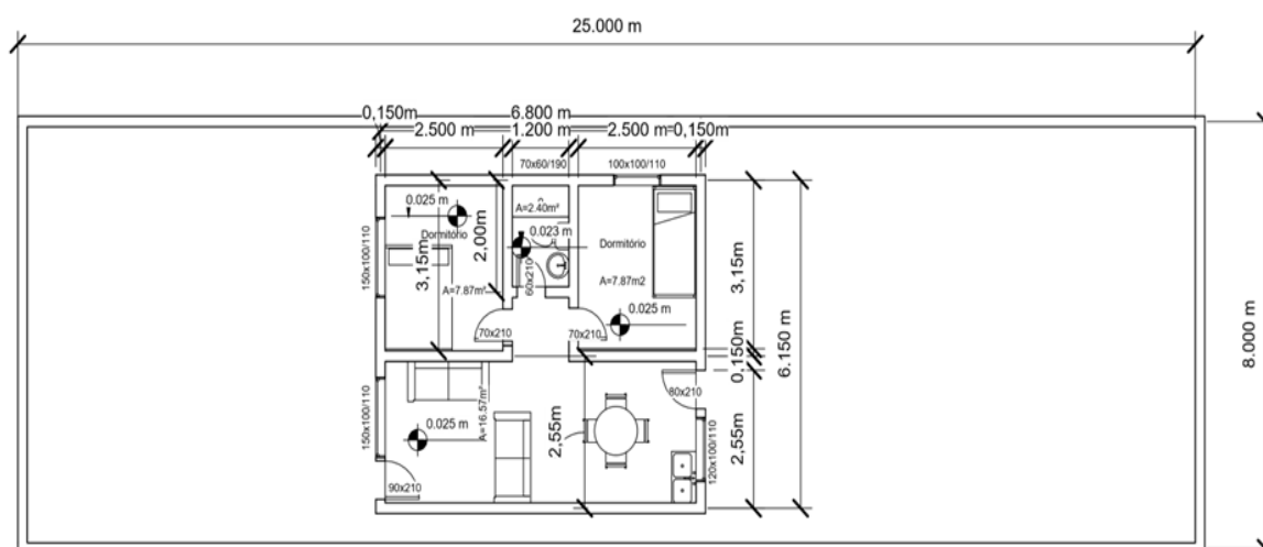
FIGURA 2. Planta baixa da casa antes da reforma realizada.
