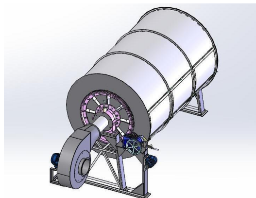
FIGURA 1. Diagrama esquemático do sistema no software SolidWorks.
