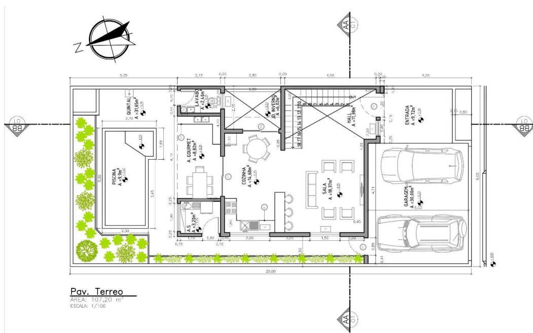
FIGURA 1. Planta Baixa Pavimento Térreo.
