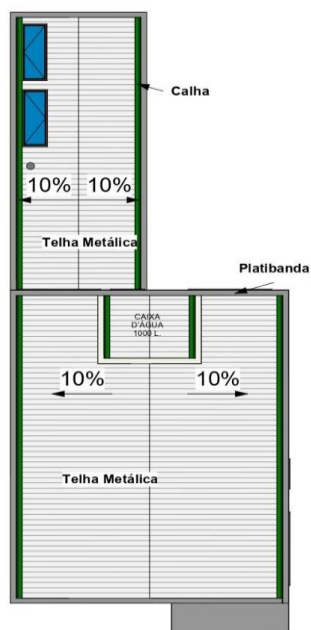
FIGURA 3. Planta Baixa de Cobertura
