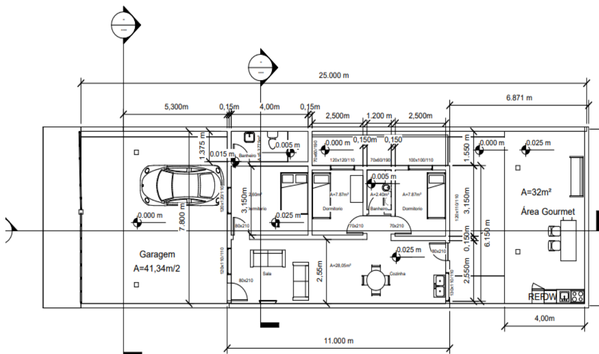
FIGURA 3. Planta baixa da casa após a reforma.
