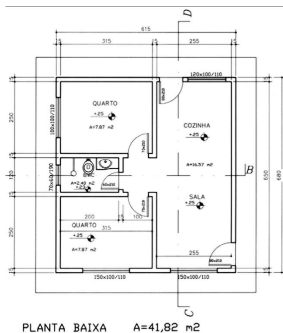
FIGURA 1. Planta baixa disponibilizada em sala de aula.
