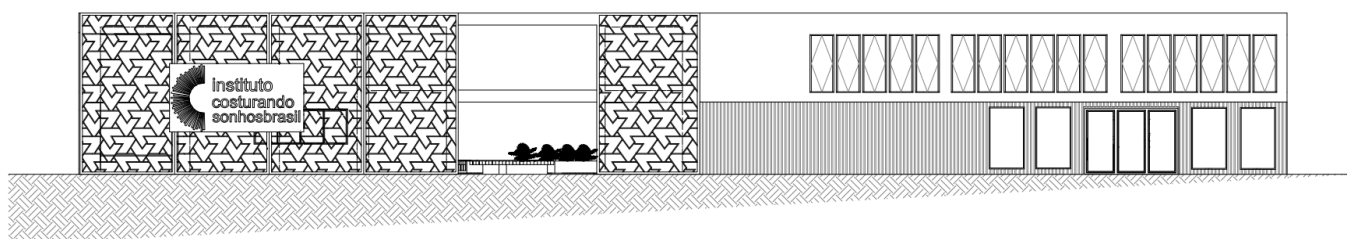
FIGURA 5. Elevação 1 do Projeto Costurando Sonhos Brasil.
