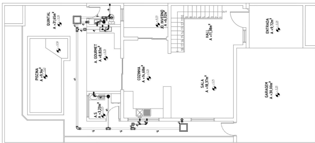
FIGURA 11. Planta Hidrossanitária Esgoto Pavimento Térreo FONTE: José Walter, 2024.
