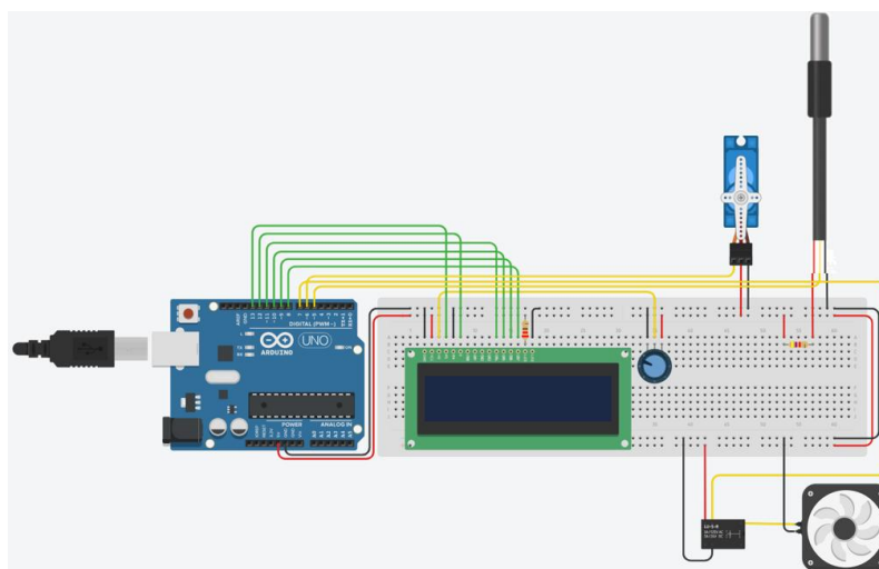
FIGURA 2. Diagrama esquemático eletrônico do protótipo na ferramenta TinkerCAD.
