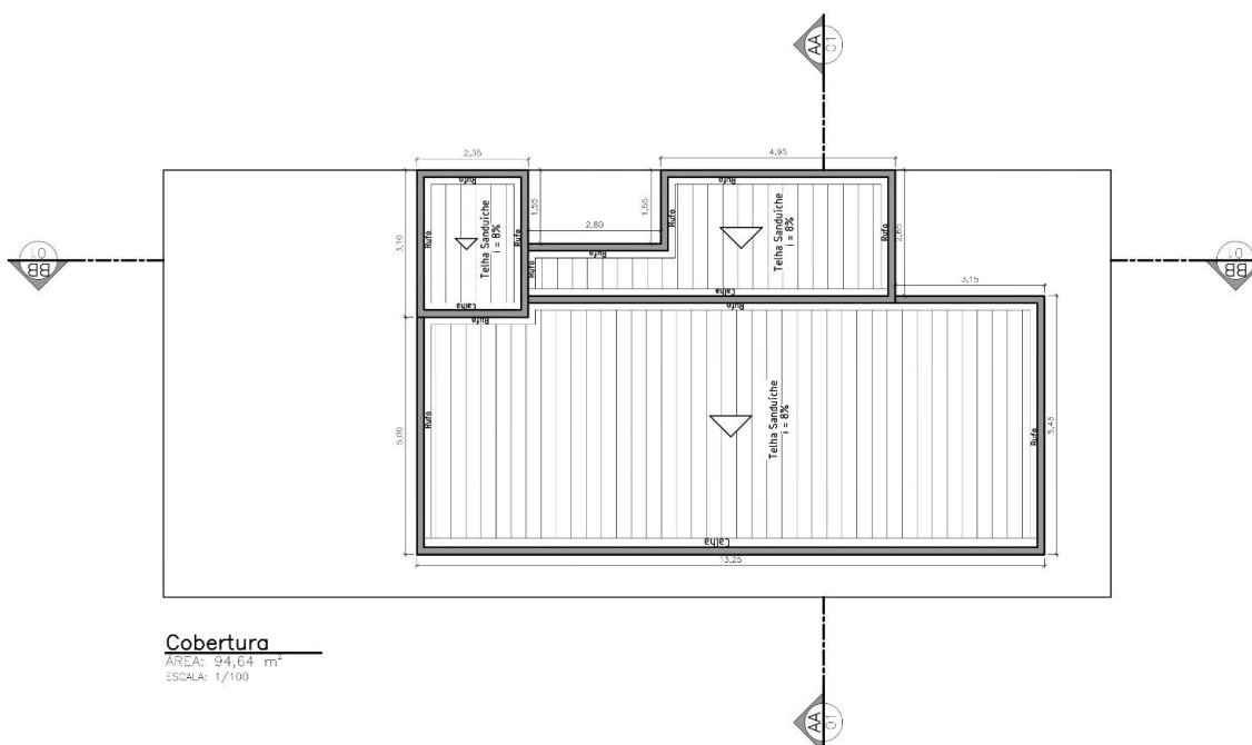
FIGURA 3. Planta Baixa Cobertura.
