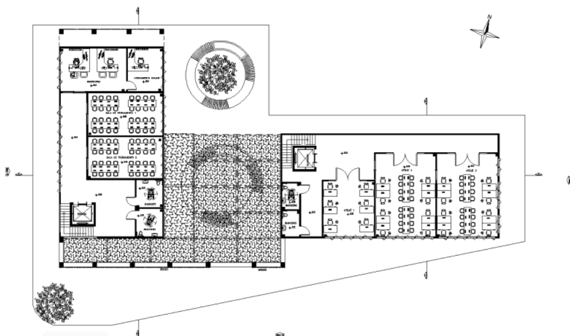
FIGURA 4. Planta - Pavimento 2 do Projeto Costurando Sonhos Brasil.
