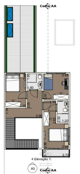
FIGURA 2. Planta Baixa Primeiro Pavimento
