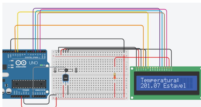
FIGURA 01. Foto do sensor de temperatura, à esquerda, e sensor de gás à direita, no TinkerCad.
