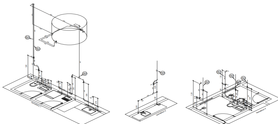
FIGURA 8. Planta Isométrica hidrossanitário Água Fria
