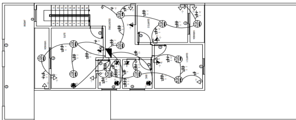
FIGURA 7. Planta Elétrica
