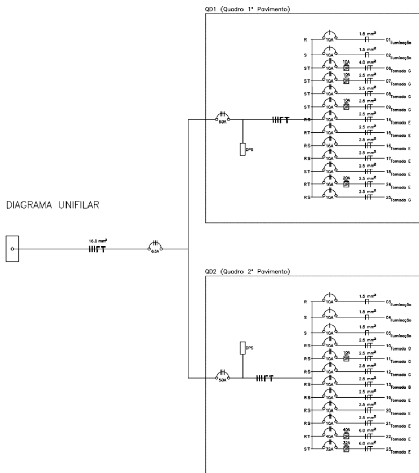
FIGURA 8. Diagrama Unifilar Projeto Elétrico FONTE: José Walter, 2024.
