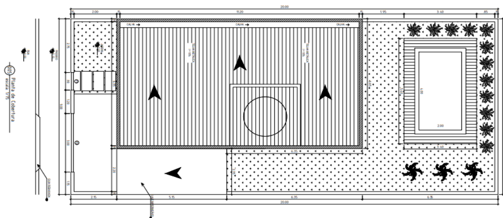
FIGURA 3. Planta Baixa Cobertura.
